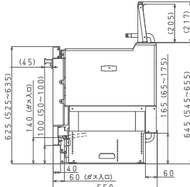
図は高さ850mmキッチン枠 (750~860mm設置可能)
