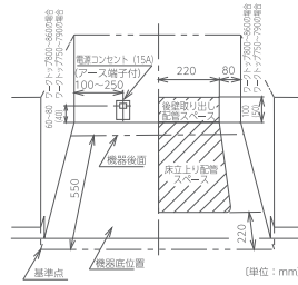
ガス配管・電源コンセント取り出し位置図 (単位: mm)
